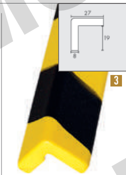
3 PGE320S - paracolpi lunghezza 780 mm x larghezza 27 mm, peso 135 gr con biadesivo PGE320SM - come sopra ma magnetico
