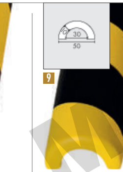
9 PGE435S - paracolpi lunghezza 780 mm x altezza 30 mm, peso 135 gr con biadesivo
