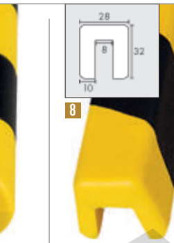
8 PGE230S - paracolpi lunghezza 780 mm x larghezza 28 mm, peso 135 gr senza biadesivo
